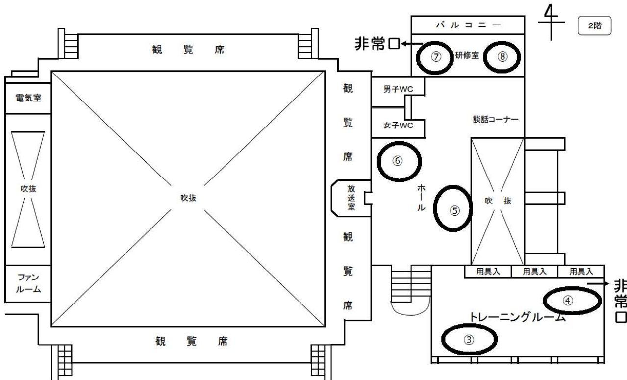
2階平面図
